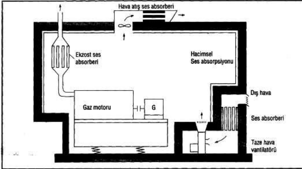
Şekil 7: Bölgesel ve lokal ısı kuvvet santrali (CO-GENERATION) için ses söndürme tedbirleri
