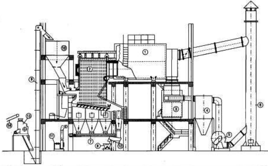
Şekil 3 : Kömür yakıtlı ön ve arka ocaklı skoç tipi buhar kazanı
