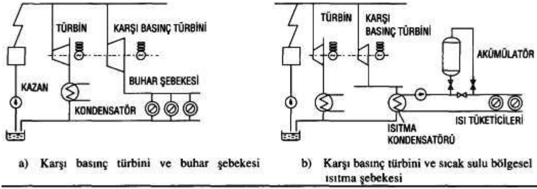
Şekil 5a : Buhar Türbinli Birleşik Enerji Santralleri
