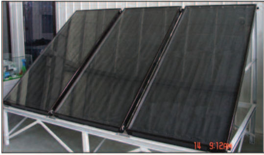
Şekil 4. Düzlem toplaçlardan oluşan ısı toplama ünitesi
