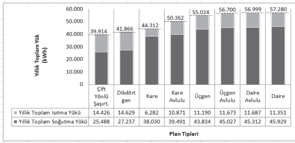
Şekil 6. Antalya İçin Hesaplanan Yıllık Isıtma ve Soğutma Yükü Değerleri
