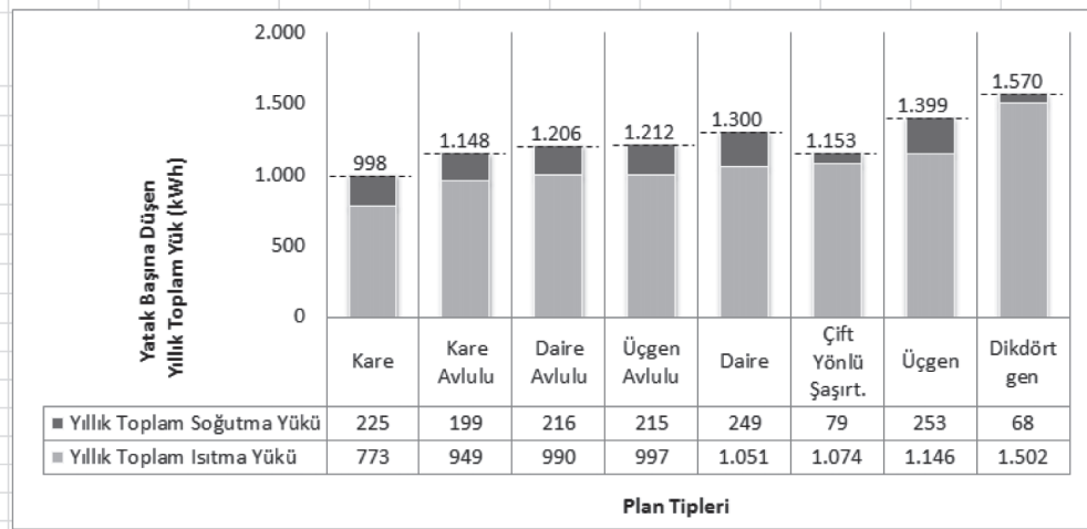
Şekil 5. İstanbul Yatak Başına Düşen Isıtma ve Soğutma Yüğü Değerleri
