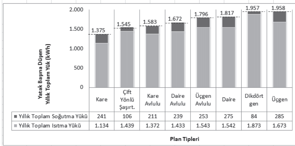
Şekil 3. Ankara Yatak Başına Düşen Isıtma Ve Soğutma Yüğü Değerleri
