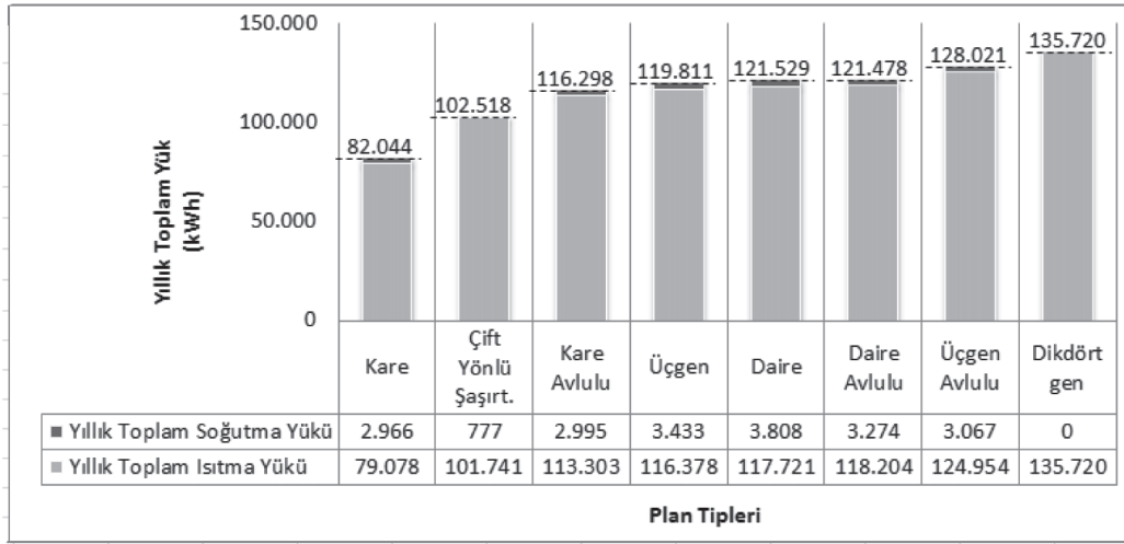
Şekil 10. Erzurum İçin Hesaplanan Yıllık Isıtma ve Soğutma Yükü Değer
