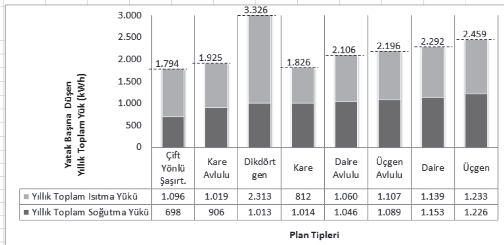
Şekil 9. Diyarbakır Yatak Başına Düşen Isıtma ve Soğutma Yükü Değerleri
