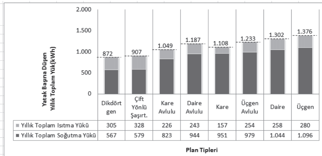
Şekil 7. Antalya Yatak Başına Düşen Isıtma ve Soğutma Yükü Değerleri
