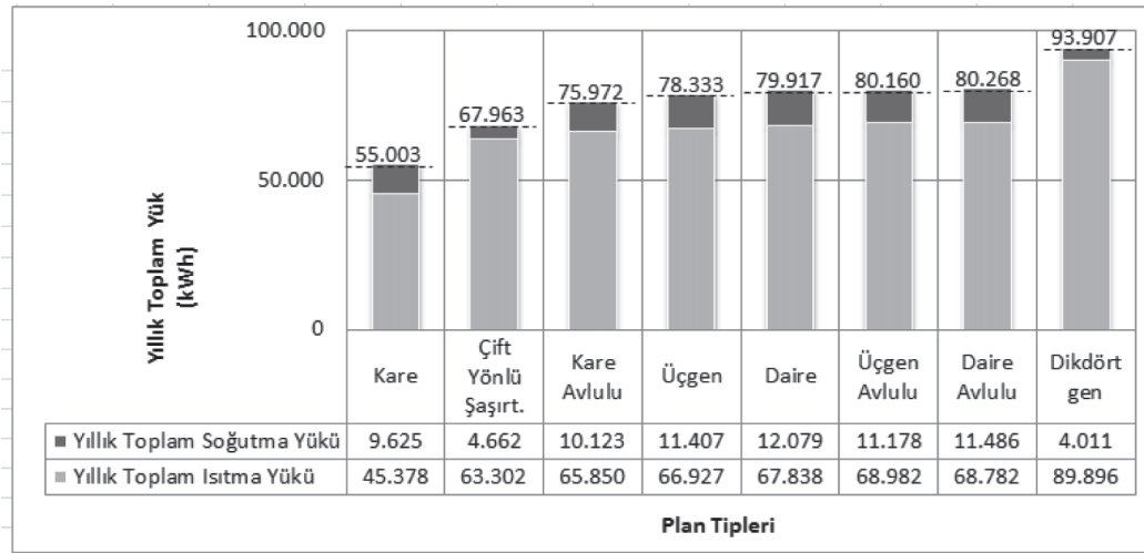
Şekil 2. Ankara İçin Hesaplanan Yıllık Isıtma ve Soğutma Yükü Değerleri
