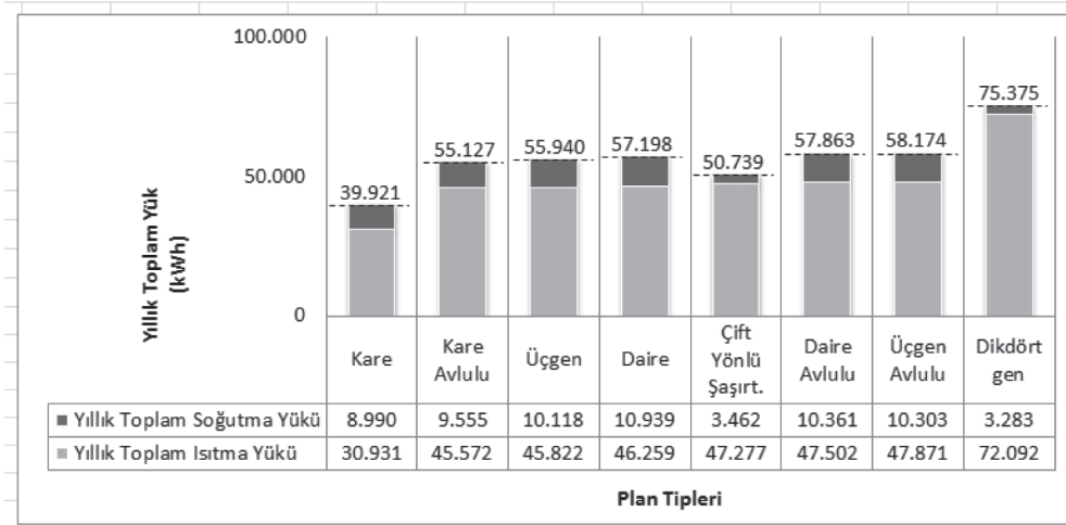
Şekil 4. İstanbul İçin Hesaplanan Yıllık Isıtma ve Soğutma Yüğü Değerleri
