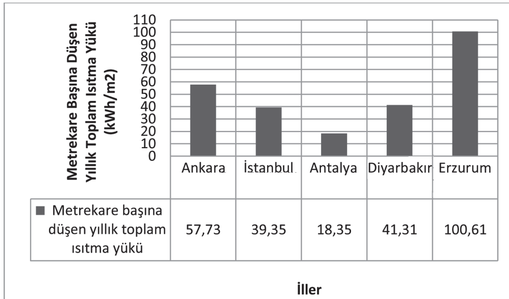
Şekil 12. En Verimli Plan Tiplerinin Metrekare Başına Düşen Yıllık Toplam Isıtma ve Soğutma Yükü Değerleri
