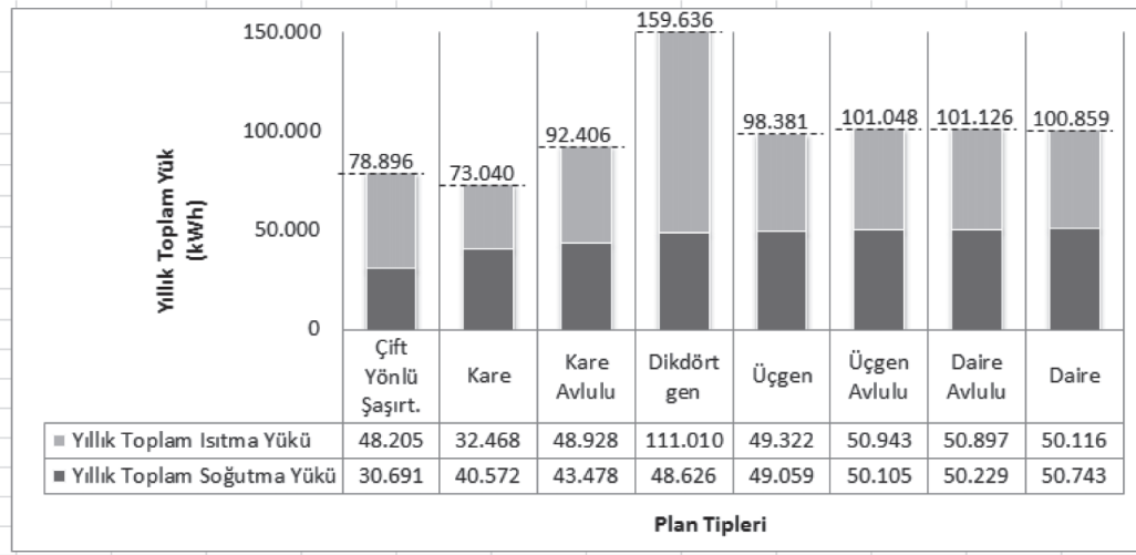
Şekil 8. Diyarbakır İçin Hesaplanan Yıllık Isıtma ve Soğutma Yükü Değerleri
